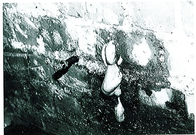
Injectienippel met kraan zijn in de lekkende muur geplaatst. De injectie-pomp en -slang kunnen nu worden aangesloten.
